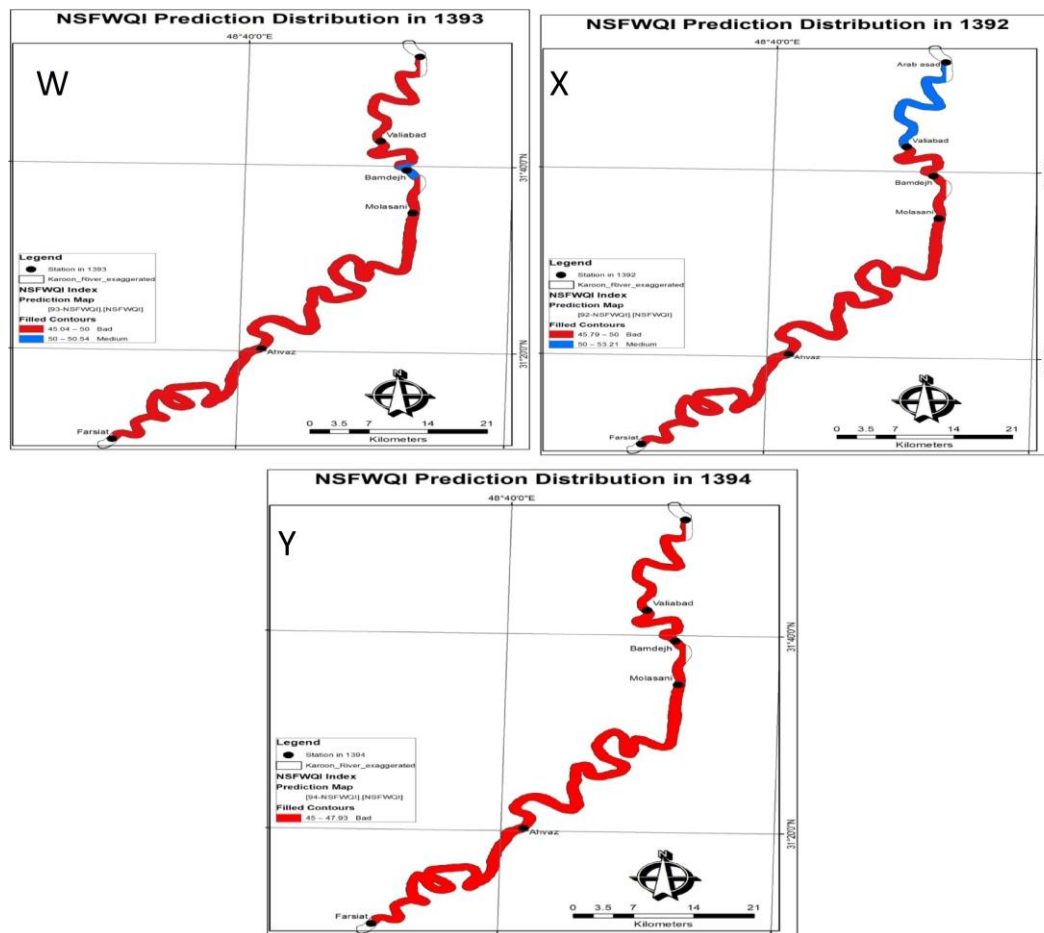
شکل ۷- (X) پهنه‌بندی شاخص کیفیت آب بازه رودخانه کارون NSFQI در سال ۱۳۹۲ (Y) رودخانه کارون NSFQI در سال ۱۳۹۴ (W) پهنه‌بندی شاخص کیفیت آب بازه رودخانه کارون NSFQI در سال ۱۳۹۲
