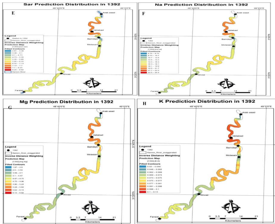
شکل ۳- (E) پهنه‌بندی مقادیر نسبت جذب سدیم (F) پهنه‌بندی درصد عنصر سدیم (G) پهنه‌بندی عنصر منیزیم (H) پهنه‌بندی عنصر پتاسیم
