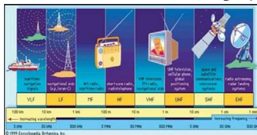
شکل ۱. طیف امواج الکترومغناطیسی با کاربری های مختلف
