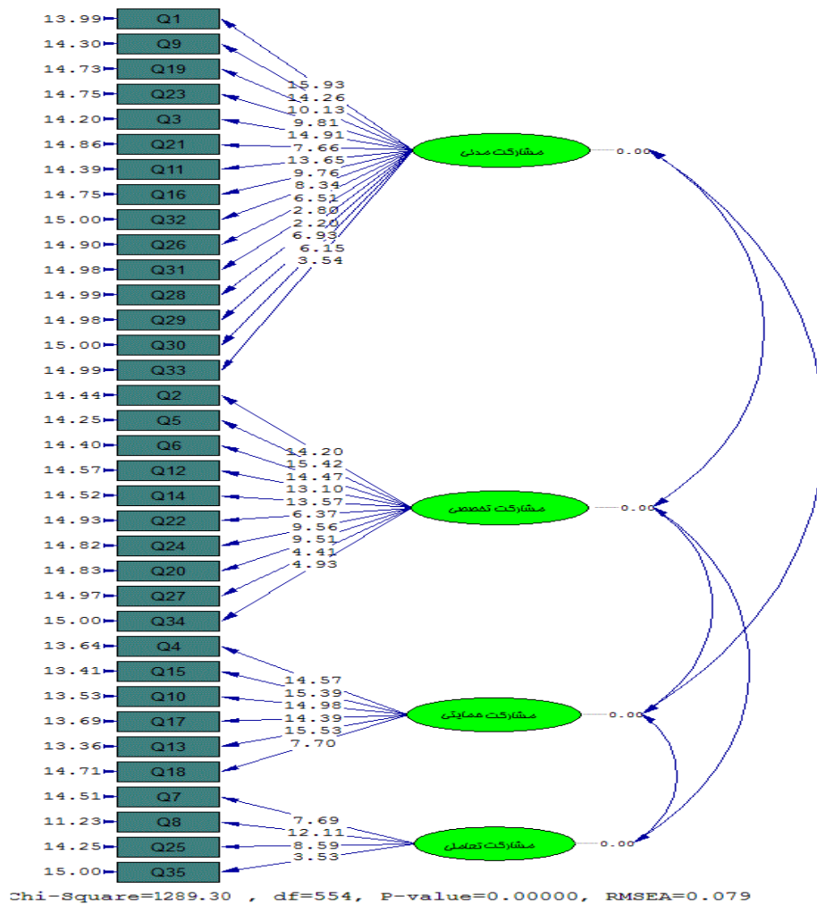
شکل ۱- مقادیر برآورد شده بارهای عاملی
