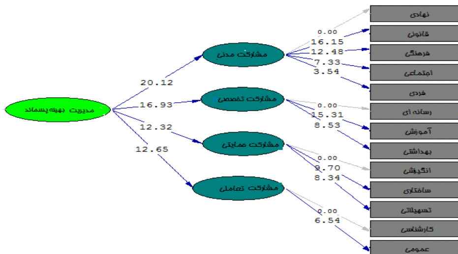
شکل ۳- خروجی مدل برازش مولفه ها
