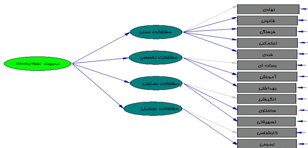
شکل ۲- مدل مفهومی ارتباط بین عوامل تعریف شده
